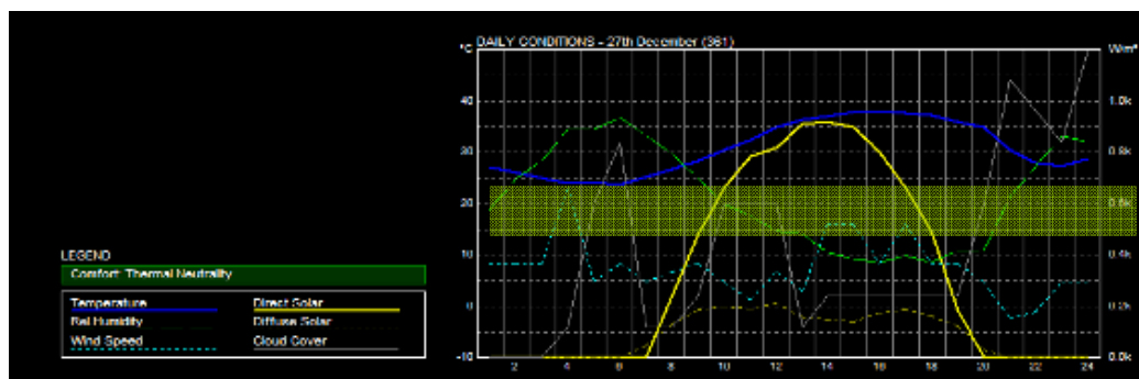
Gráfico. 5. Temperatura, humedad, Velocidad del viento, radiación solar directa y difusa para un día de temperatura pico en verano. Fuente Elaboración propia con software ECOTEC.
